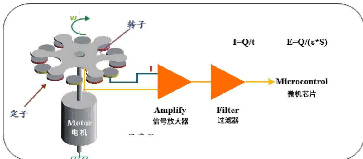
场磨式大气电场仪测量原理模型
